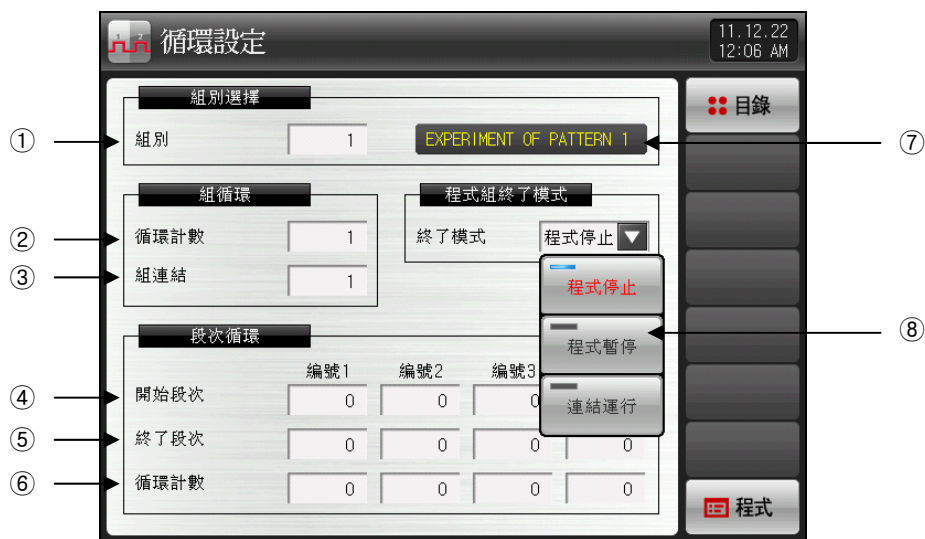
[图5-3] 定式及片段循环设定画面
