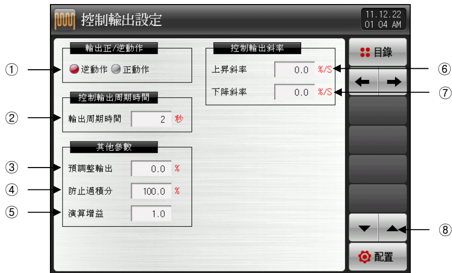
[图12-5]输出设定第2画面
