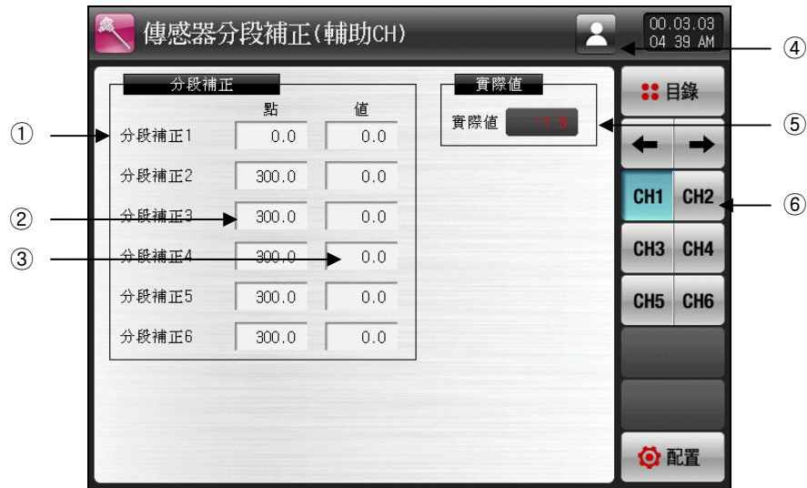
[图22-7] 辅助频道每区间传感输入补正画面-1
