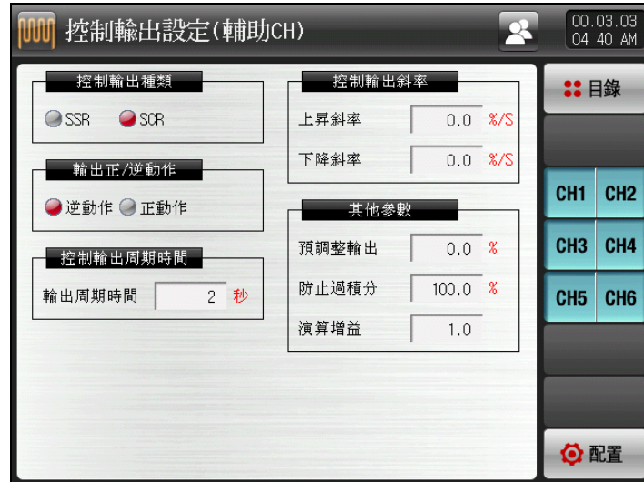
[图22-10] 辅助频道控制输出设定画面-2
