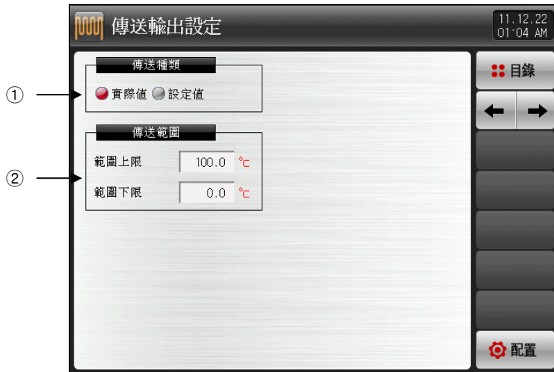
[图12-6] 输出设定第3画面(PV, SP设定的时候)
