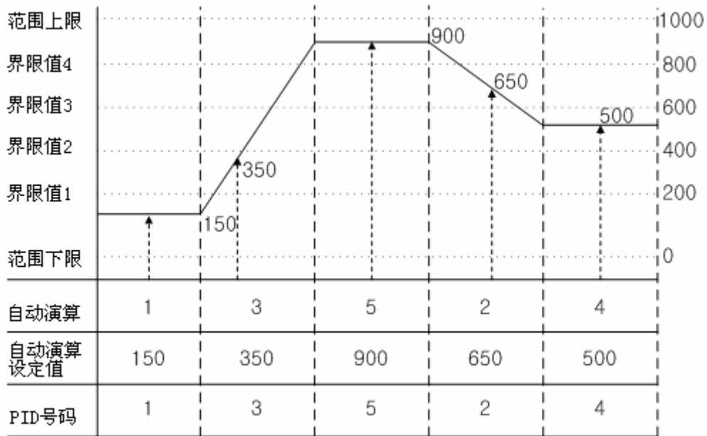
程式运行 自动演算(分区)
