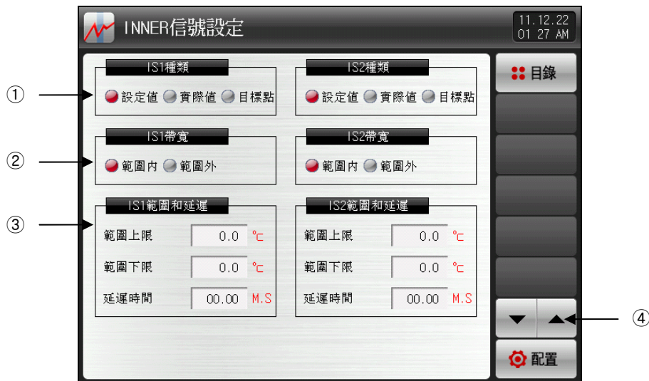
[图15-1]内部信号设定第1画面
