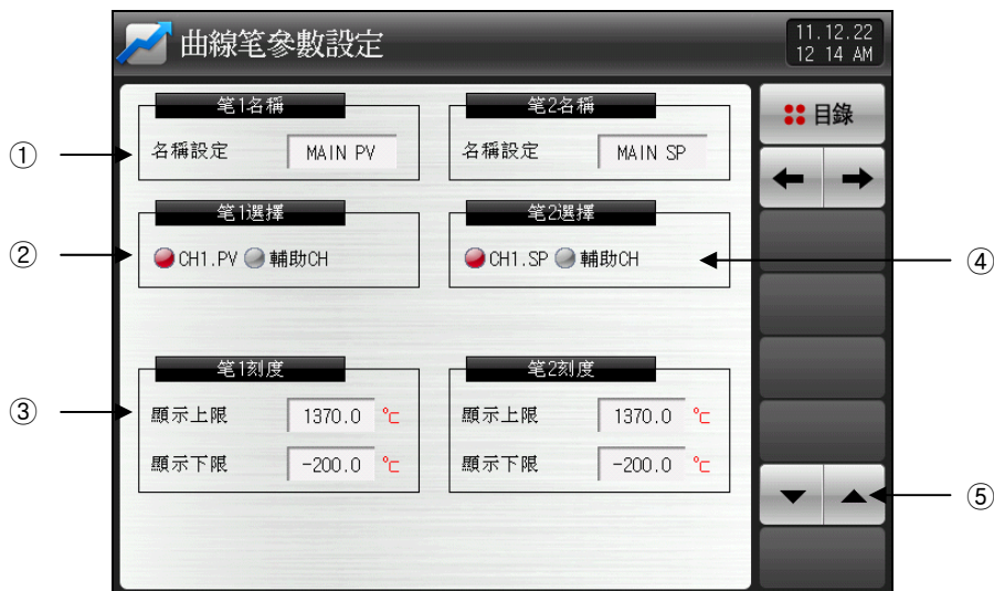
[图6-9] 曲线图&amp;保存设定第4画面-1
