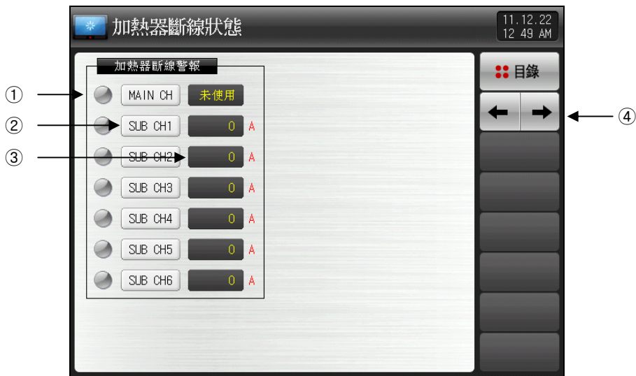
[图7-4] 加热器断线状态画面
