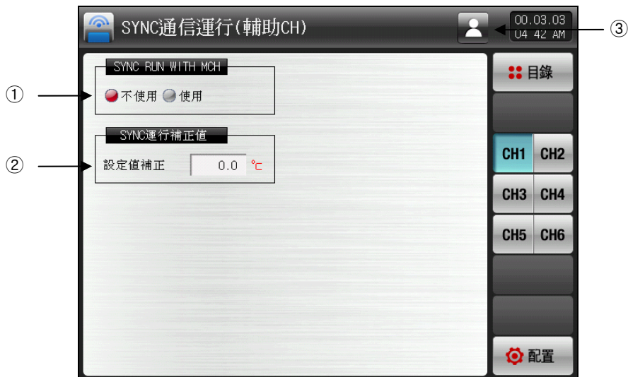
[图22-13] 辅助频道通讯设定画面-1
