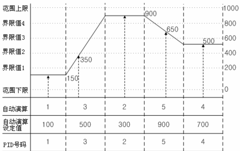
程式运行 自动演算 (区域)
