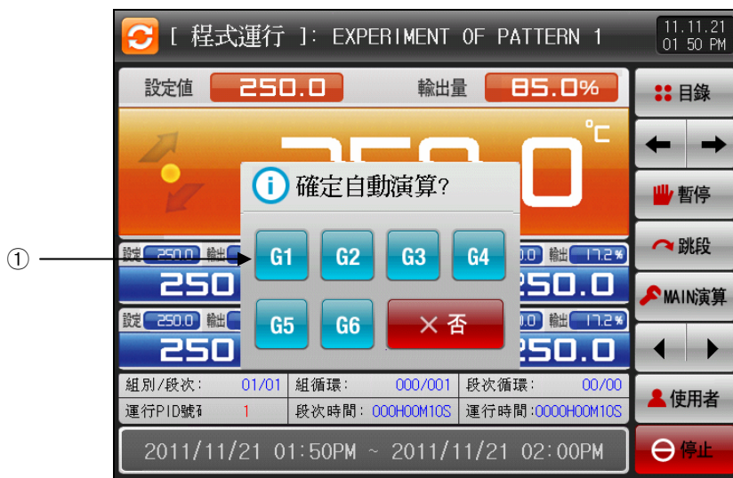
[图3-17]分区PID自动演算画面
