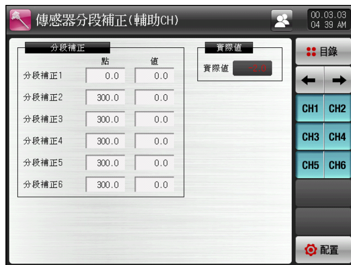
[图22-8] 辅助频道每区间传感输入补正画面-02
