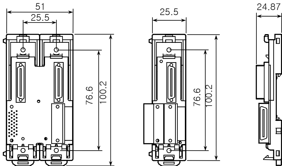
主单位 BACK COVER
