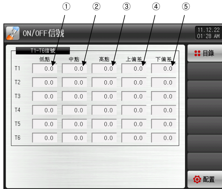
[图16-1]ON/OFF信号设定画面
