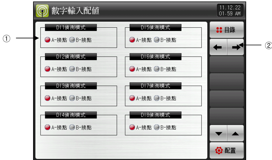
[图19-2]DI功能及动作设定第二画面
