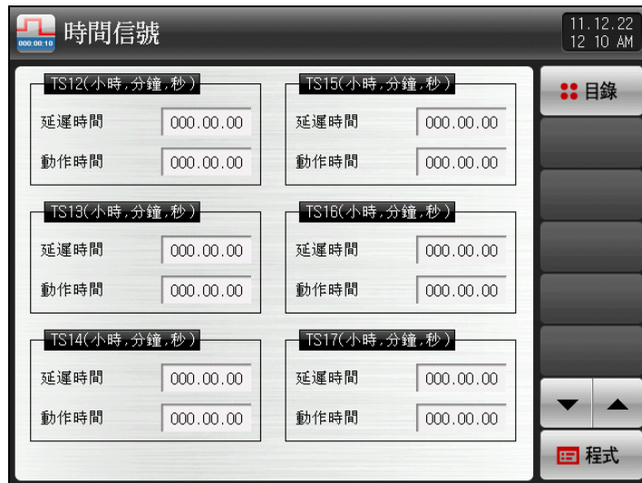
[图5-8] 时间信息 设定第3画面
