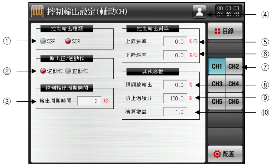
[图22-9]辅助频道控制输出设定画面-1
