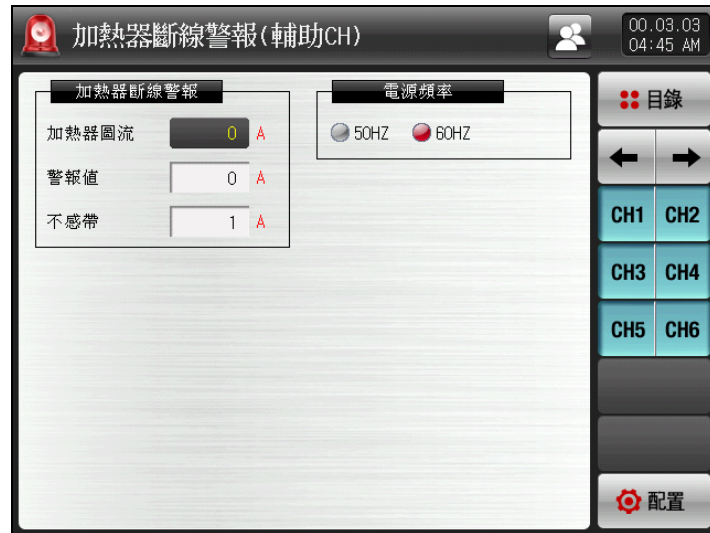
[图22-21] 加热器断线报警信号设定画面-2
