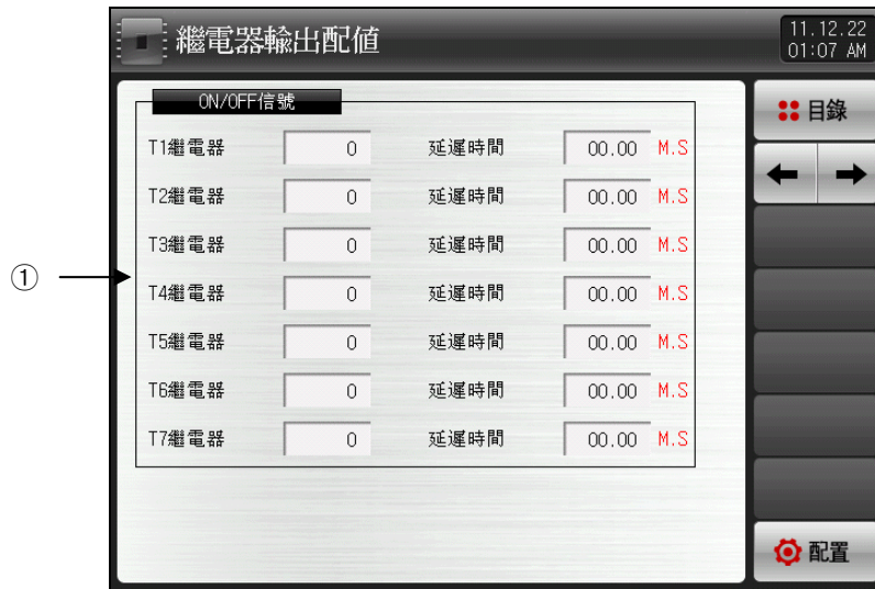
[图13-3] ON/OFF信号继电器设定画面
