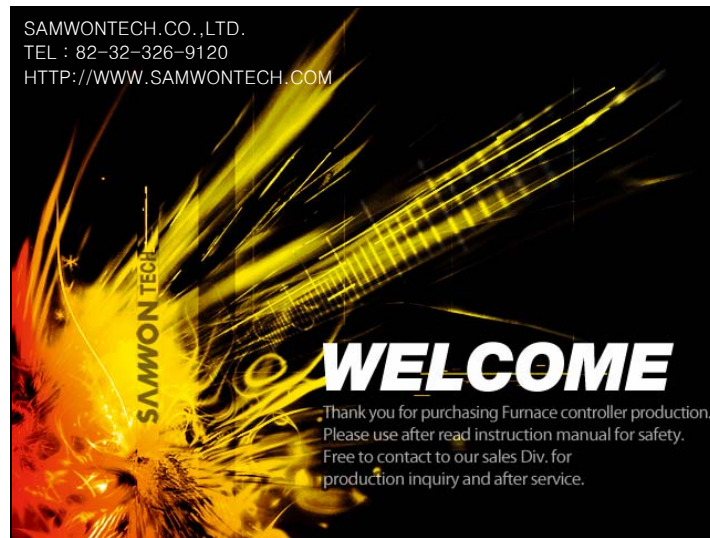
[图21-4] 初始画面-1
