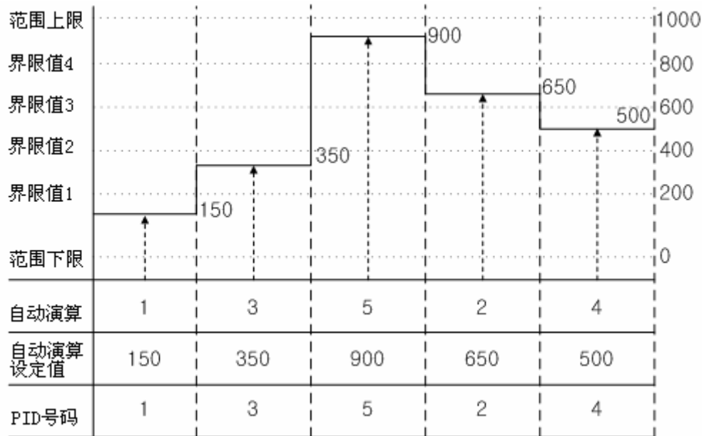
停止运行 自动演算(分区)
