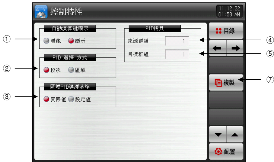
[图18-2]PID适用范围设定第二画面
