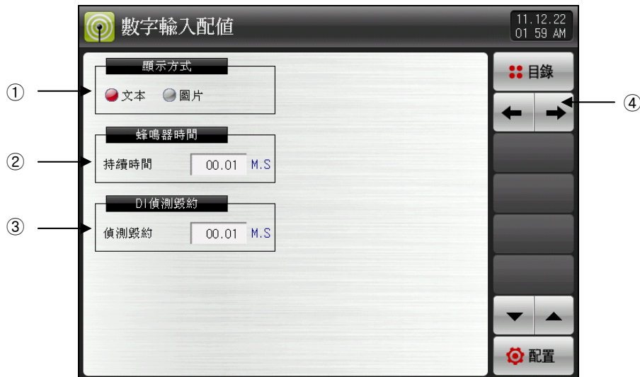
[图19-1]DI功能及动作设定第一画面
