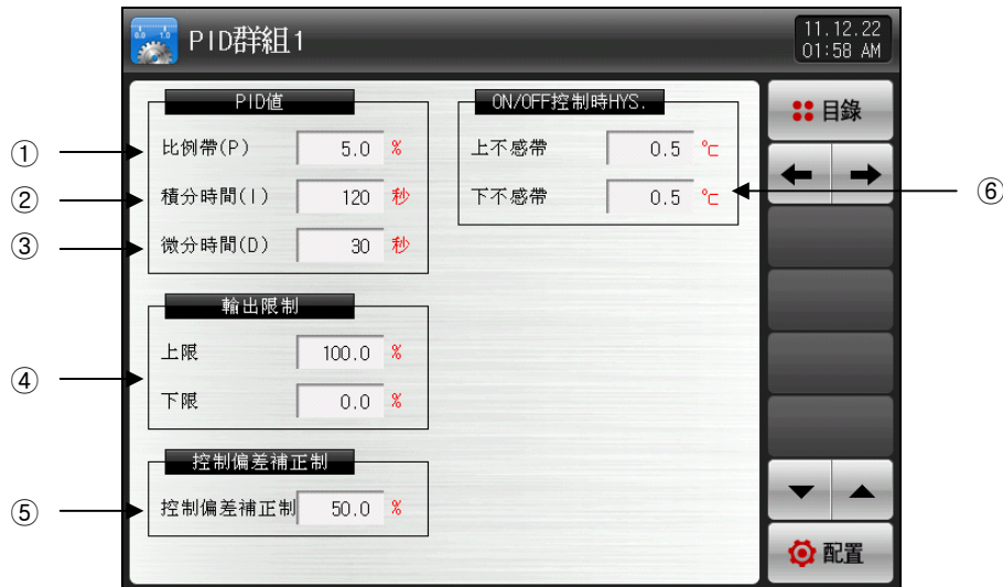
[图18-3]PID组合设定画面
