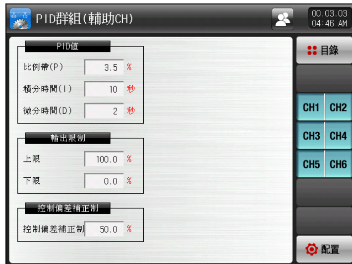
[图22-23] 辅助频道PID组合设定画面-2
