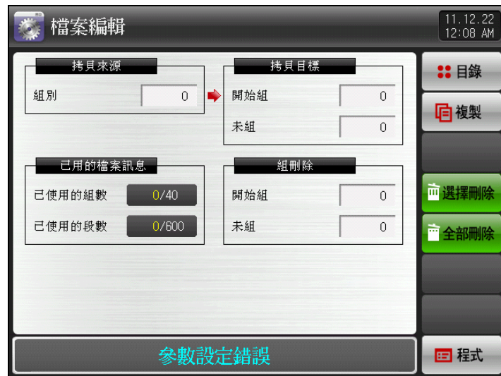
[图5-5] 文件编辑画面-2
