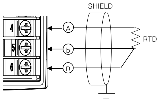
(一) 测温电阻体输入(RTD INPUT)
